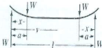
Gambar 2.2. Balok sesudah terjadi deformasi
