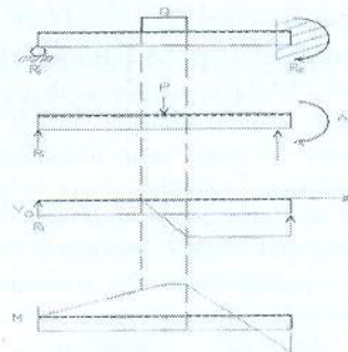
Gambar 2.4. Diagram gaya geser dan diagram momen tumpuan jepit dan rol.
