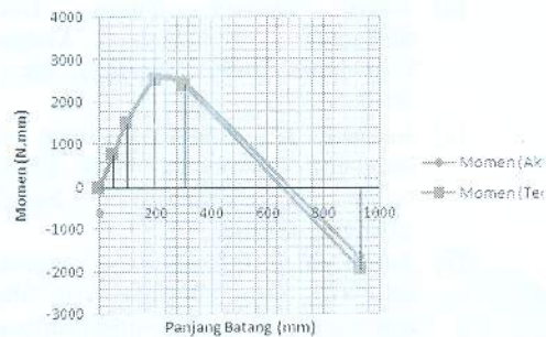
Gambar 4.14 Grafik diagram momen batang pada beban 22,2687 N & Jarak a = 200 mm
