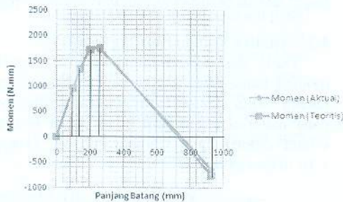
Gambar 4.8 Grafik diagram momen batang pada beban 13,145 N & Jarak a = 200 mm
