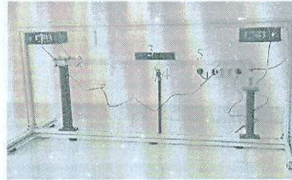
Gambar 3.3. Mesin uji defleksi batang lentur
