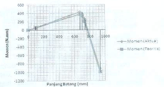
Gambar 4.7 Grafik diagram momen batang pada beban 6,573 N & Jarak a = 700 mm
