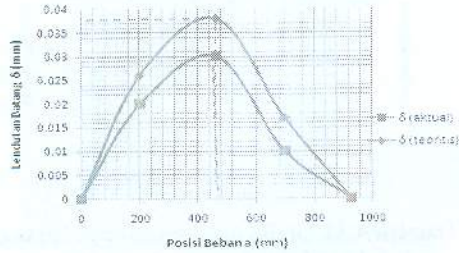
Gambar 4.1 Grafik lendutan batang lentur \delta (mm) pada pembebanan 6,573 N
