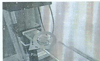
Gambar 2.3. Strain gauge pada tumpuan jepit
