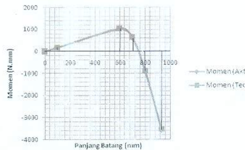
Gambar 4.16 Grafik diagram momen batang pada beban 22,2687 N & Jarak a = 700 mm
