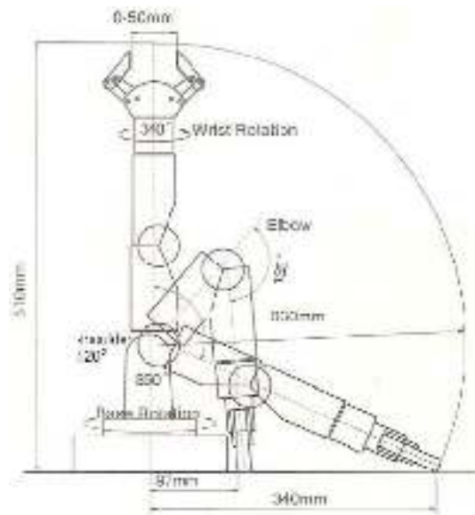
Gambar 2.1 Contoh Pergerakan Lengan Robot
