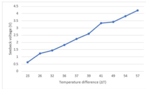
Fig. 14. Seebeck voltage.
