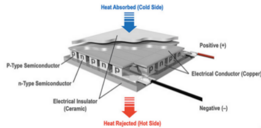
Fig. 3. TEG module [15].
